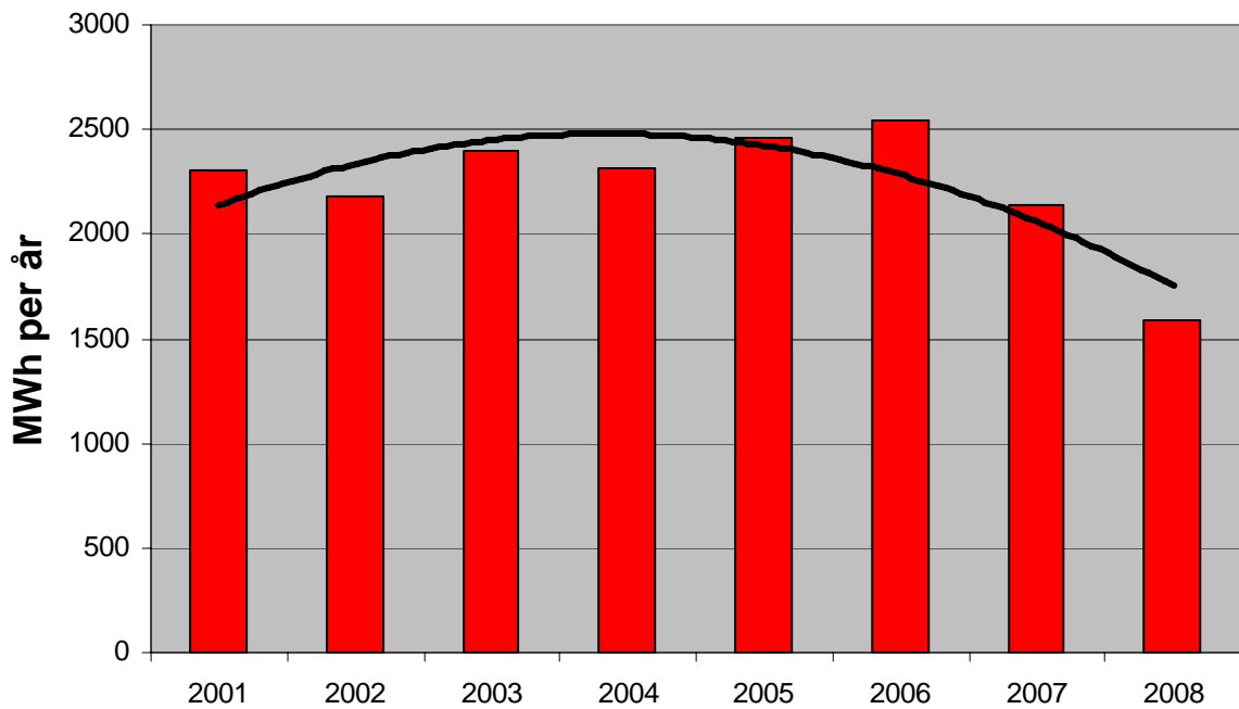
Energi för uppvärmning vid Naturbruksgymnasiet Dingle
